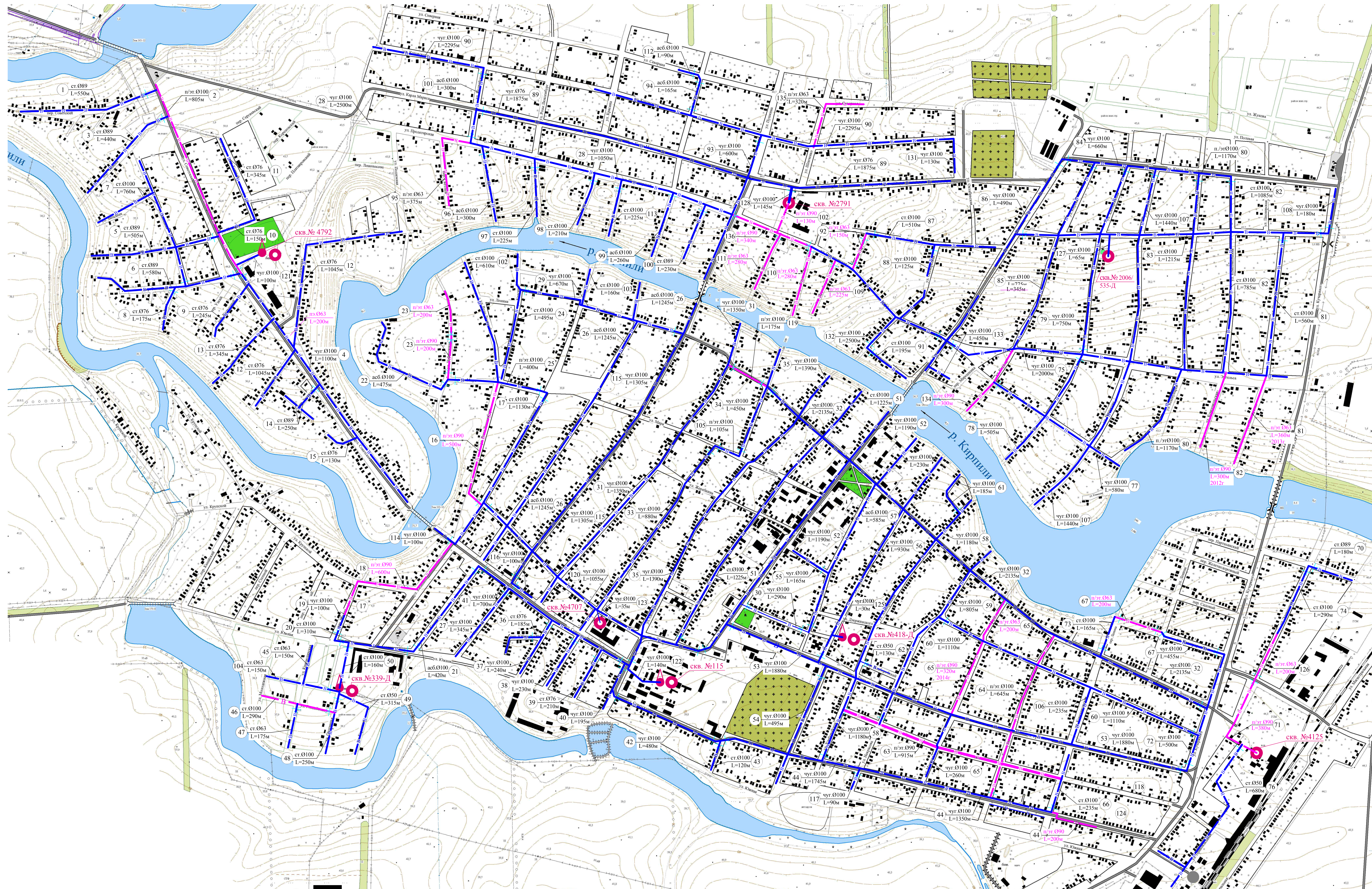
Ведомость существующих трубопроводов водоснабжения
